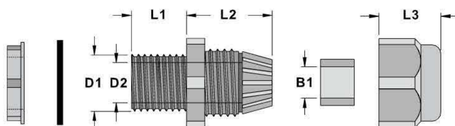
ロックナット AGL ワッシャー AGW 本体 AGB ツメ AGN シール AGS
